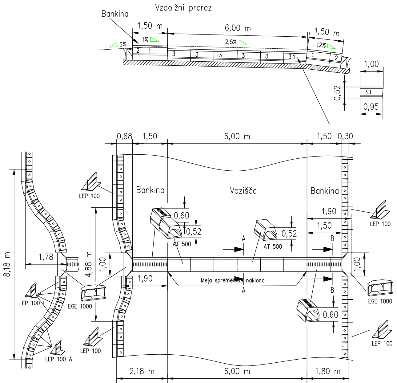
DETAJL VGRADNJE PREHODA ZA DVOŽIVKE IN VODILNIH PREGRAD
